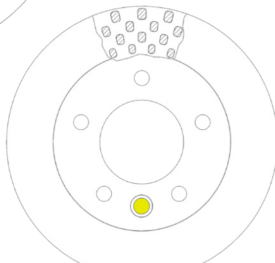
Tarcza hamulcowa z otworem do dużych śrub mocujących
