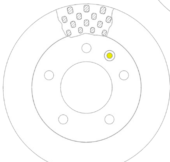
Tarcza hamulcowa z otworem do małych śrub mocujących
